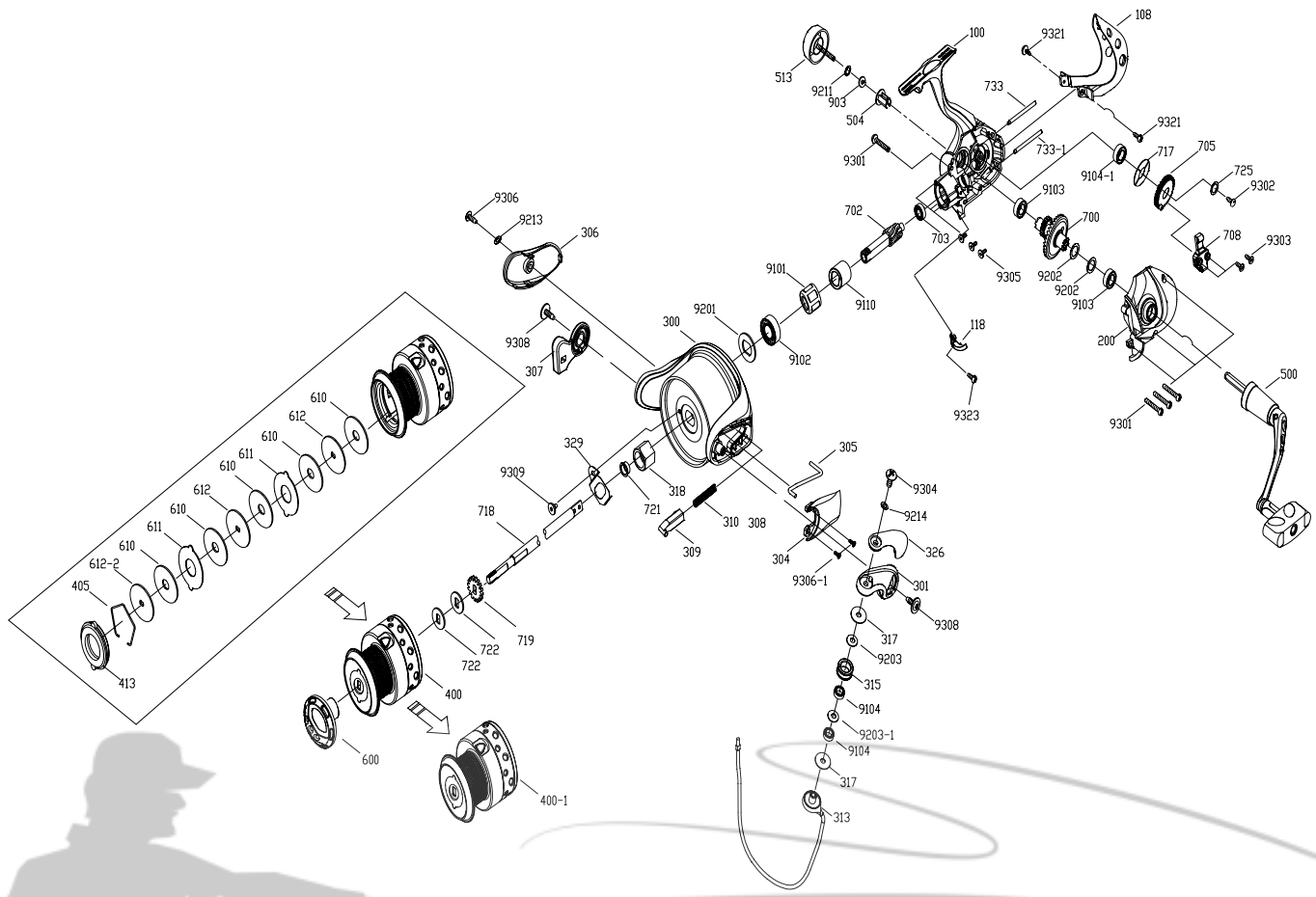
AL - 80 Spare Parts
