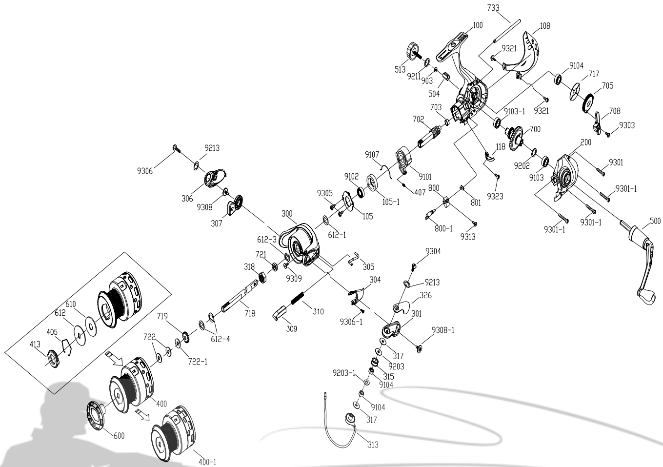
AL - 20 Spare Parts
