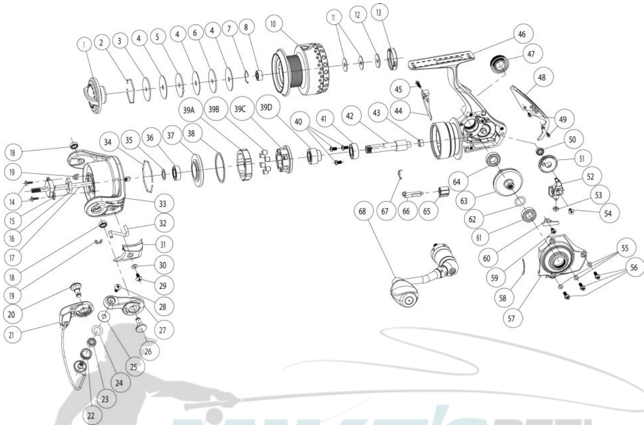
Quantum Energy E10PTIB Spinning Reel Part List
