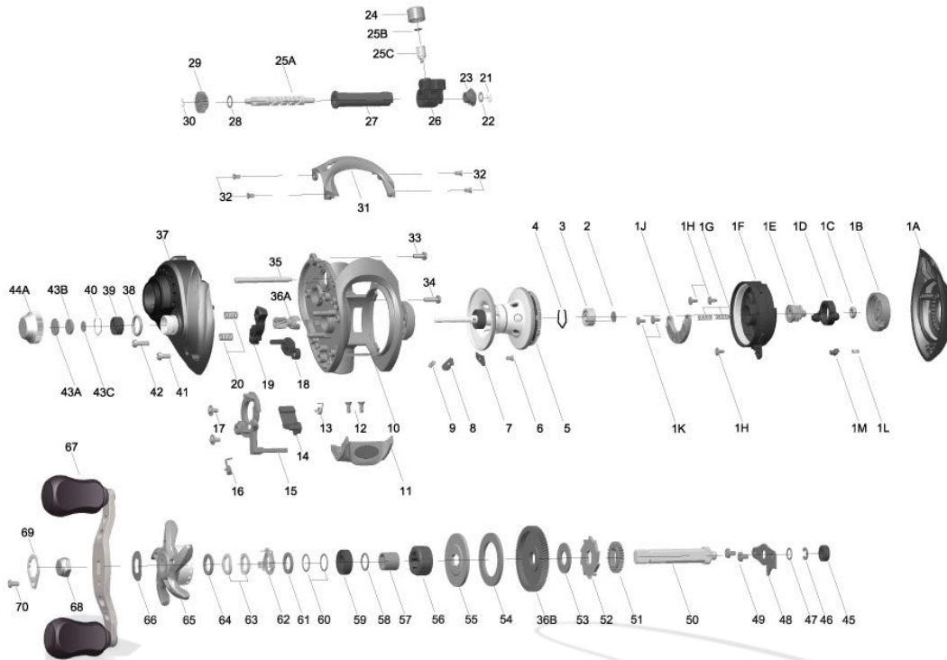
Quantum AN101H Bait Cast Reel Part List
